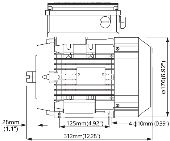
Frame Size 90L
